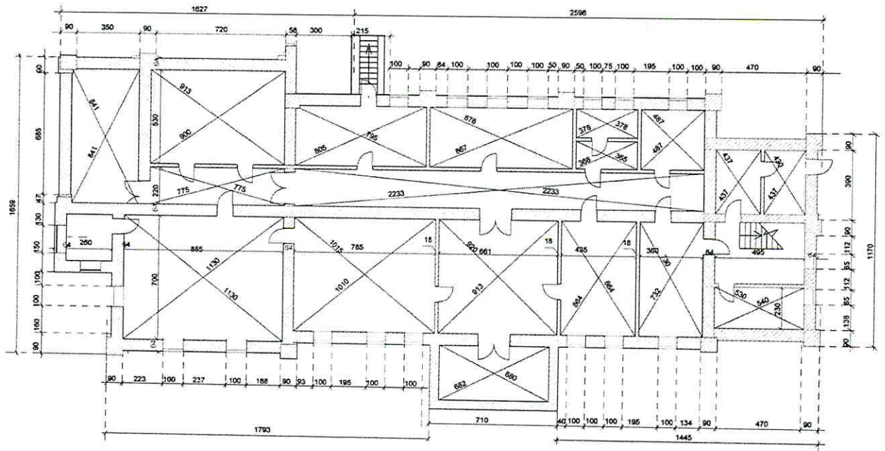
Обмерный план цокольного этажа. (Господский дом).
